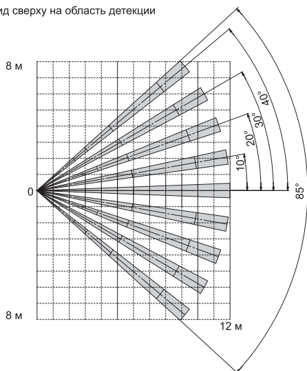
Вид сверху на область детекции
